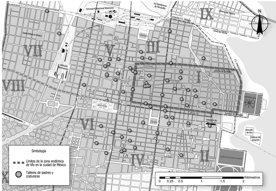
Mapa 1. Límites de la zona endémica de tifo en la ciudad de México (1920-1921)
